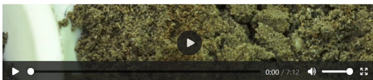
Figure 1 Beispiel für einen der 7 Böden des Dorigny-Waldes, der auf der Website präsentiert wird (screenshot von https://wp.unil.ch/swissoil/les-profiles-de-sol-de-dorigny/site-1/ ).
