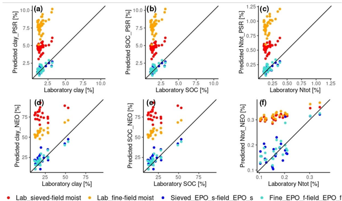
Fig. 3 Laboratoire vs. valeurs prédites des modèles cross-domain (modèle avec spectres de laboratoire, set de prédiction avec spectres de terrain) pour la teneur en argile (a et d), le carbone du sol (b et e) et l'azote total (c et f) pour le spectromètre de recherche (PSR, a-c) et le scanner (NEO, d-f). Les points de données en rouge et orange représentent les spectres non transformés, les points de données dans les tons bleus représentent les prédictions après la transformation EPO.
