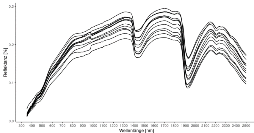
Fig. 1 Exemples de spectres de sol enregistrés in situ
